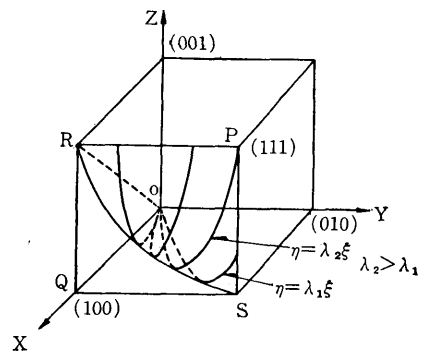
第14図 二次元集中曲面の図
