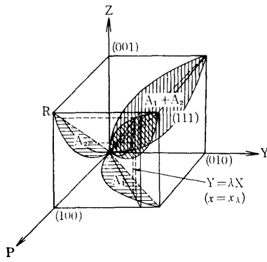
第14図 二次元集中曲面
