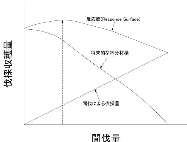
図 10. 反応面と間伐量 .
