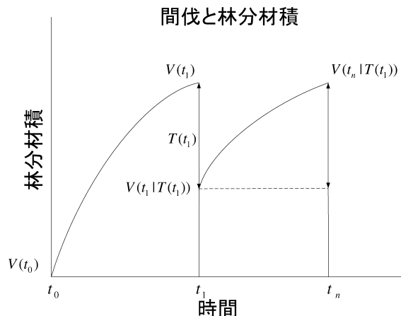
図5. 変分法と間伐戦略.
