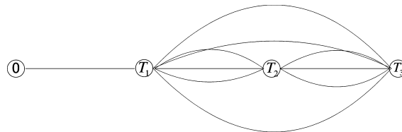
図 8. MSPATH アルゴリズムネットワーク .
