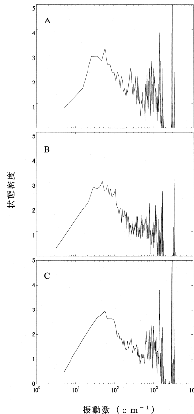
図 1. 様々な数のアミノ酸残基からなる蛋白質の基準振動の振動数毎の分布. A. クランビン(46 残基), B. エグリン \alpha (70 残基), C. ヒト・リゾチーム(130 残基).
