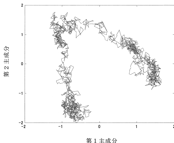
図 2. 蛋白質ヒト・リゾチームが水中で 1.0 \times 10^{-9} 秒間ゆらいでいく様子を分子動力学法で計算し、第 1・第 2 主成分軸で張られる空間内に射影したもの．第 1 主成分のゆらぎの大きさは 0.76 \text{ \AA} で、第 2 主成分のゆらぎは 0.5 \text{ \AA} でスケールしてある．
