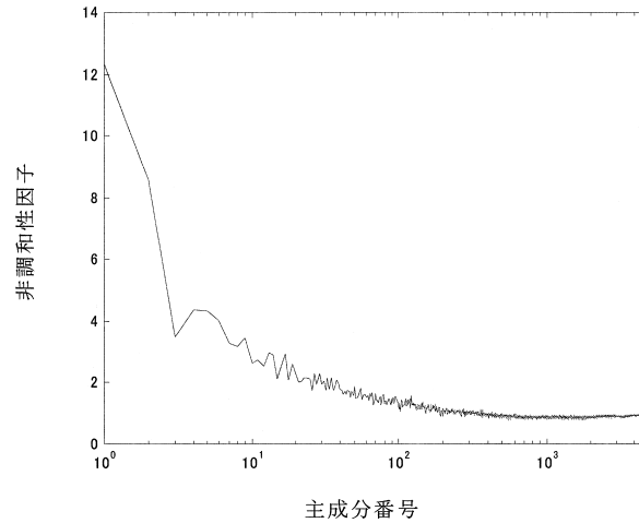
図 3. 図 2 と同じ分子動力学の結果．非調和性因子が主成分番号によってどのように変化するかを示したもの．300 番目以降では 1 に収束して非調和性がなくなっている．
