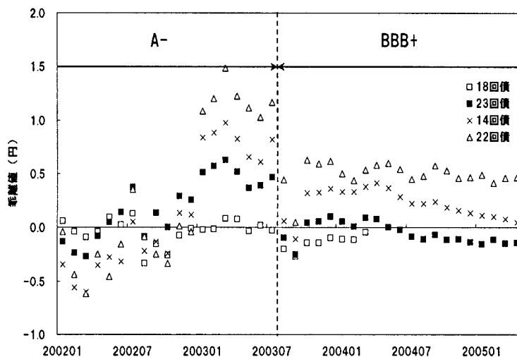
図 2. 格付け・業種の期待損失額からの乖離値の時間推移(コニカミノルタホールディングス).
