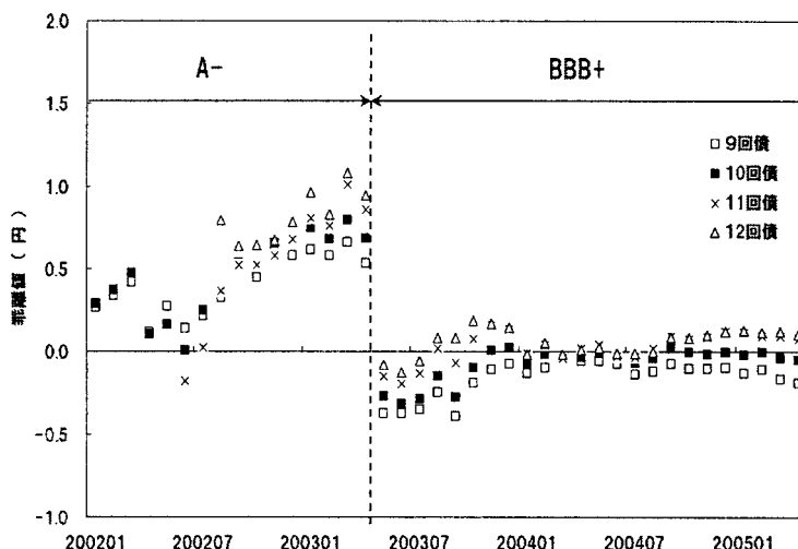
図1. 格付け・業種の期待損失額からの乖離値の時間推移(富士電機ホールディングス)。
