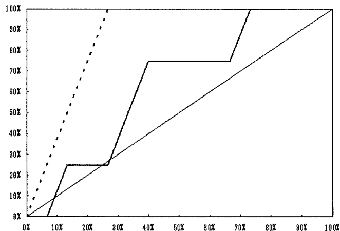
図 6. BBB+ 格付銘柄の CAP 曲線(2003 年 1 月).
