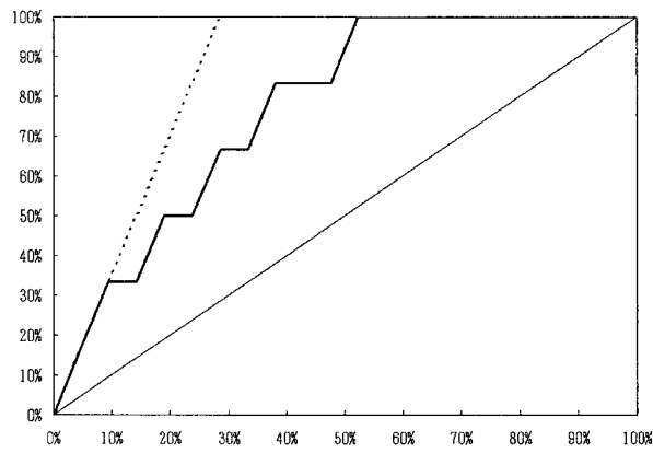
図 4. A-格付銘柄のCAP 曲線(2003年1月).
