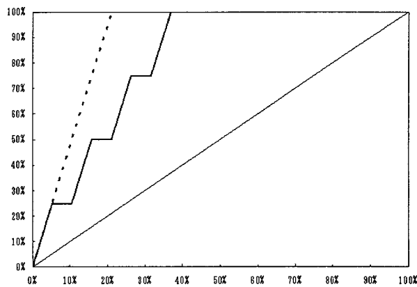
図 5. BBB+ 格付銘柄のCAP 曲線(2002年1月).
