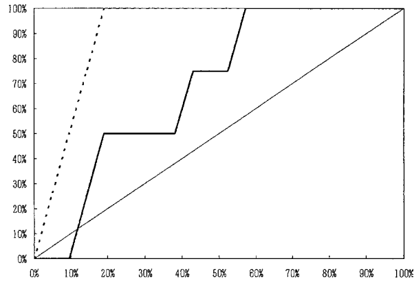
図 3. A-格付銘柄のCAP 曲線(2002年1月).
